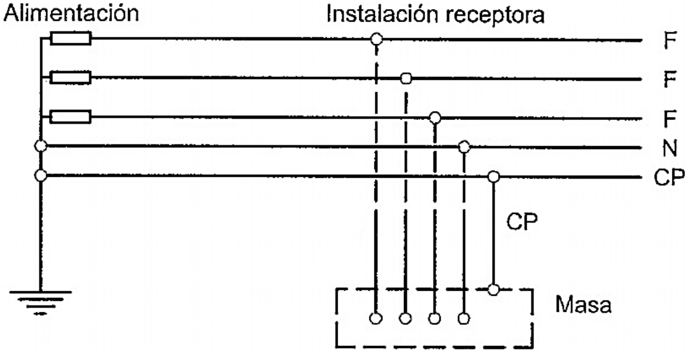
Figura 1. Esquema de distribución tipo TN-S
