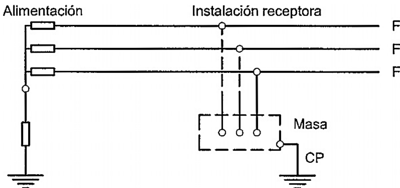
Figura 5. Esquema de distribución tipo IT
