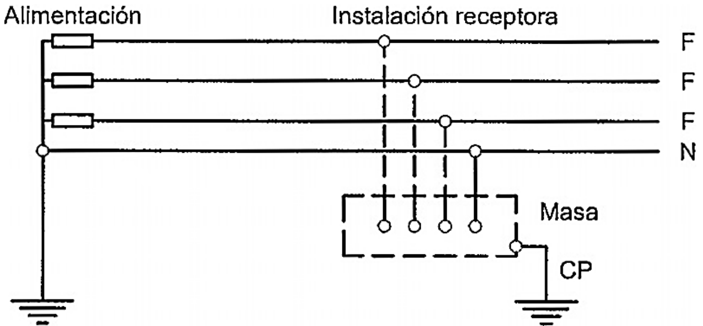
Figura 4. Esquema de distribución tipo TT
