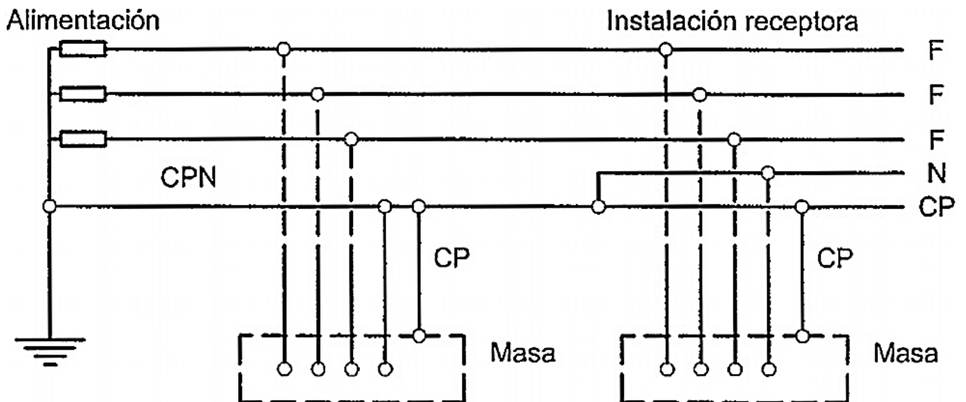
Figura 3. Esquema de distribución tipo TN-C-S
