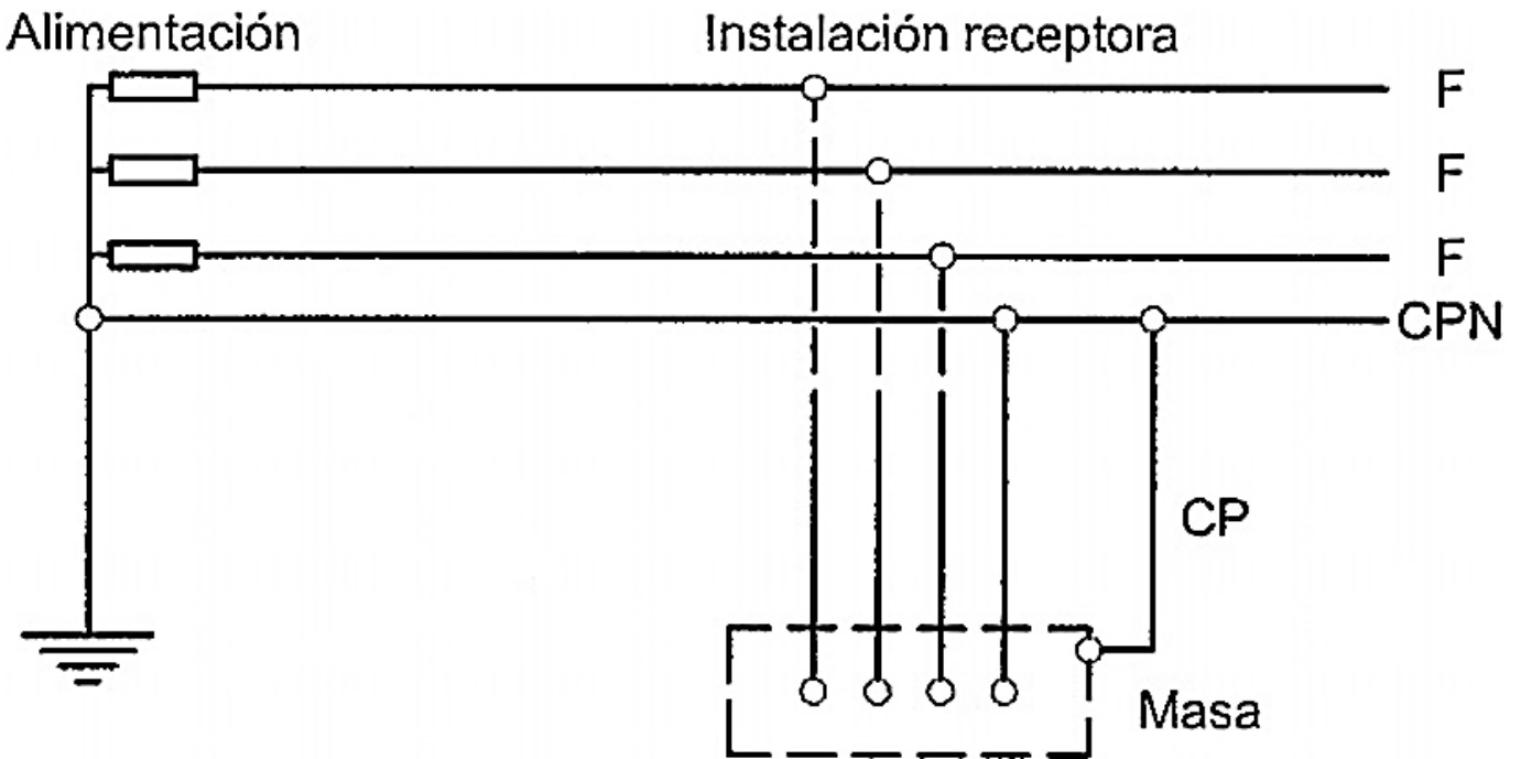
Figura 2. Esquema de distribución tipo TN-C
