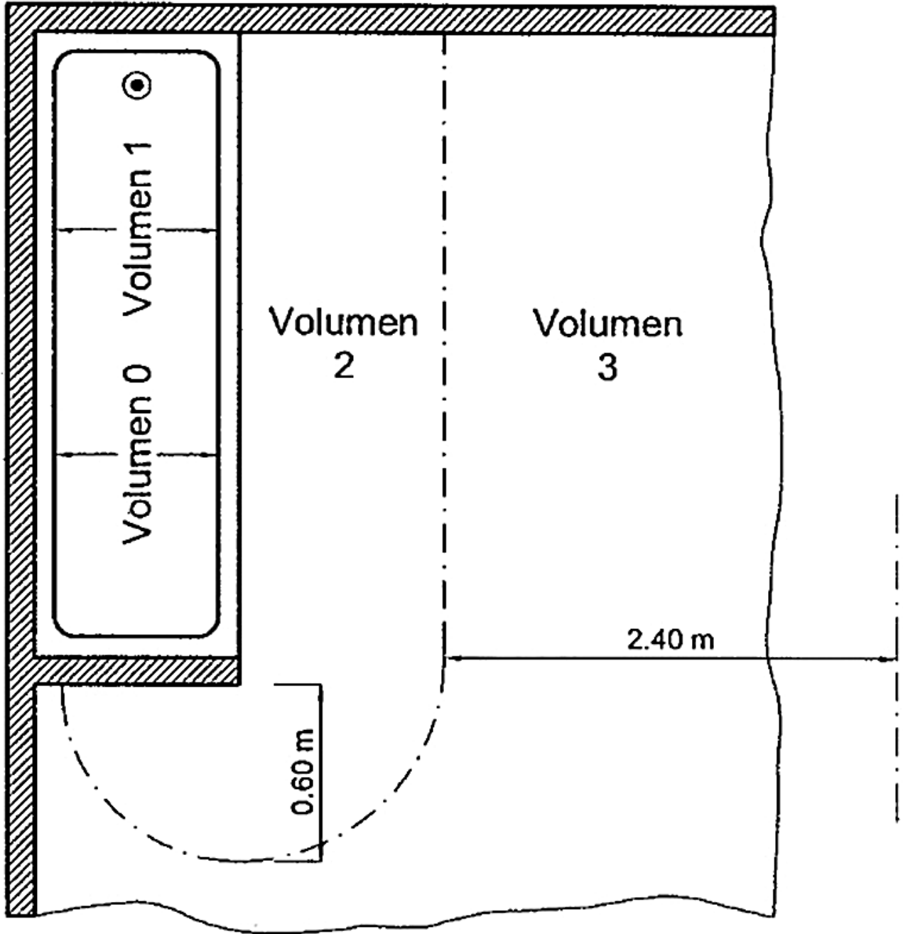
Figura 2. BAÑERA CON PARED FIJA
