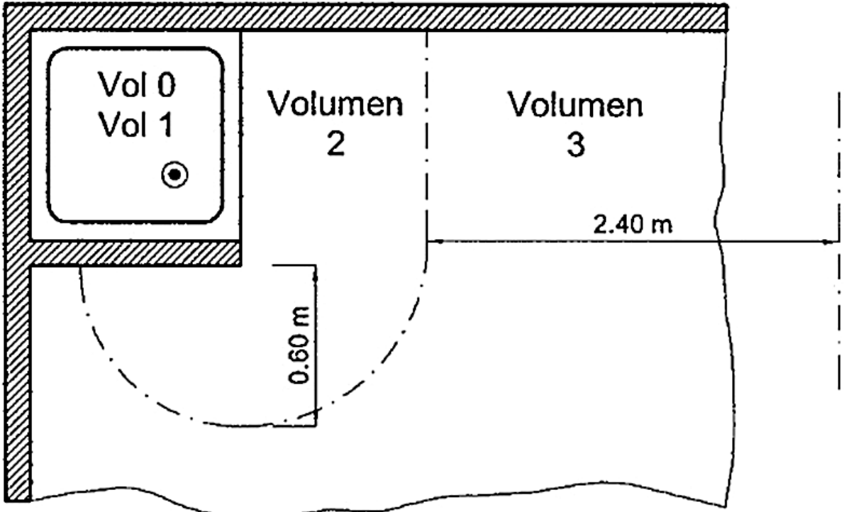
Figura 4. DUCHA CON PARED FIJA
