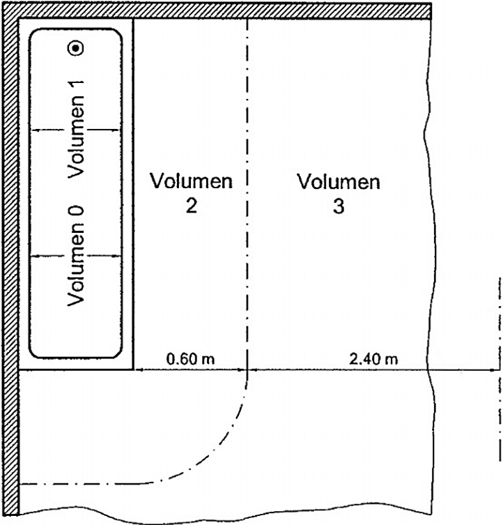
Figura 1. BAÑERA
