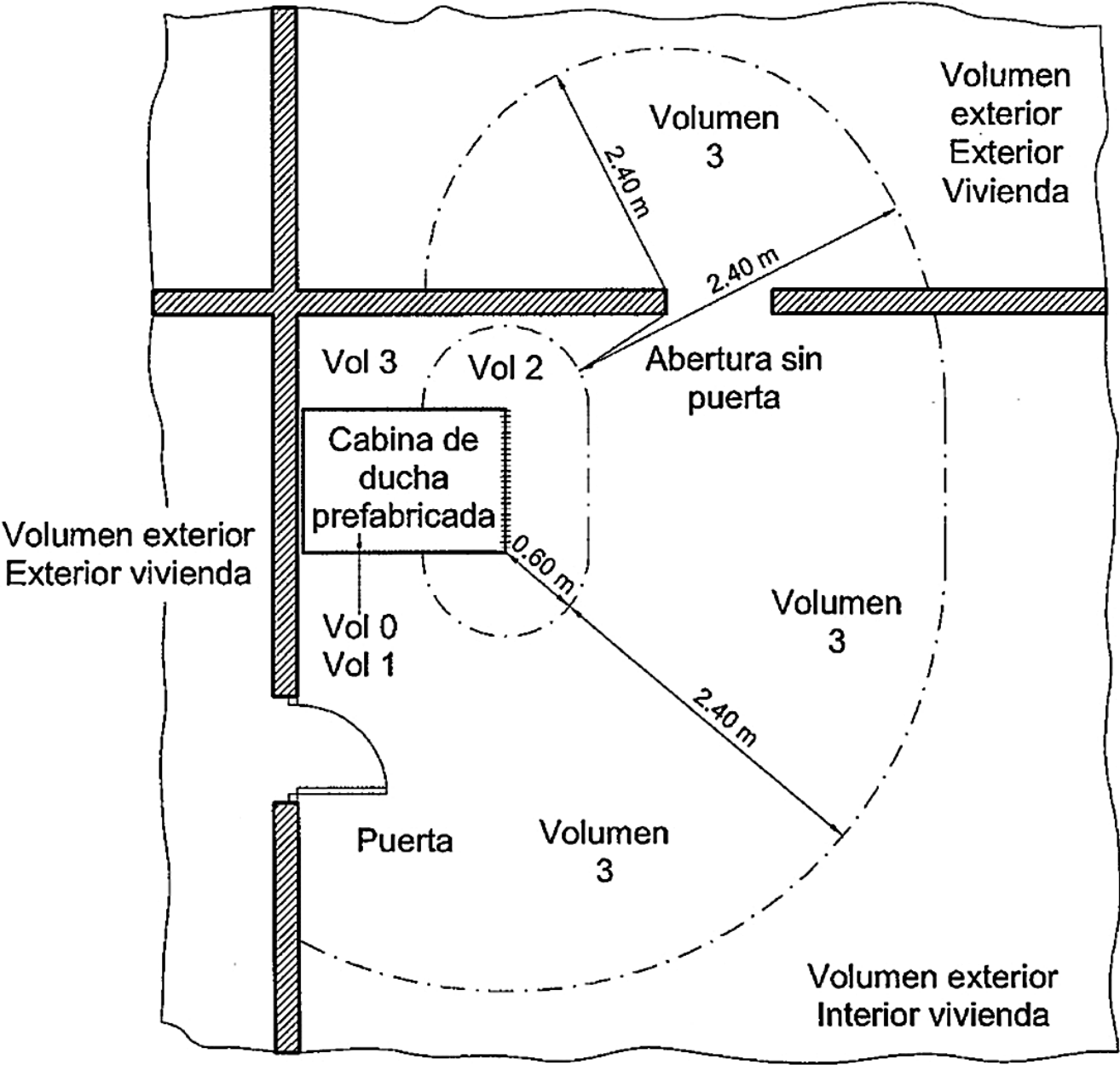
Figura 7. CABINA DE DUCHA PREFABRICADA
