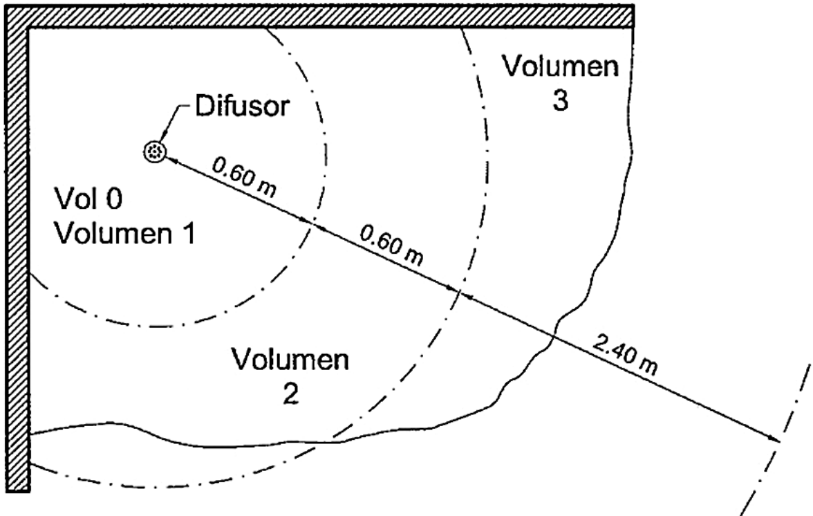
Figura 5. DUCHA SIN PLATO
