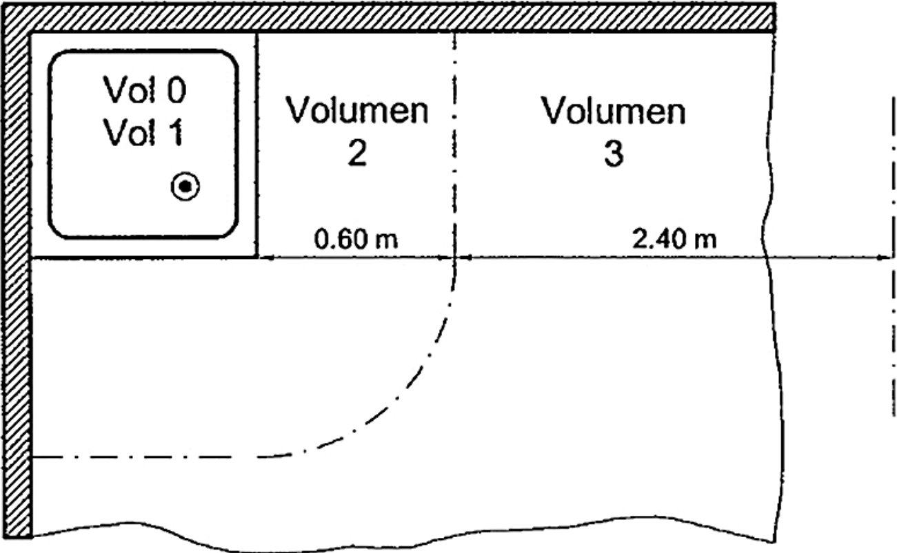
Figura 3. DUCHA
